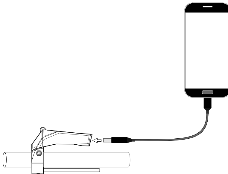
Abb. 13 USB-Anschluss
