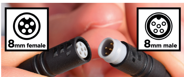
[Bild 4] Weibliche Kupplung und männlicher Stecker
